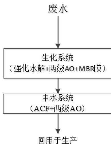
图 7.2-2 本项目依托“华星环技”生化及中水设施工艺流程图
