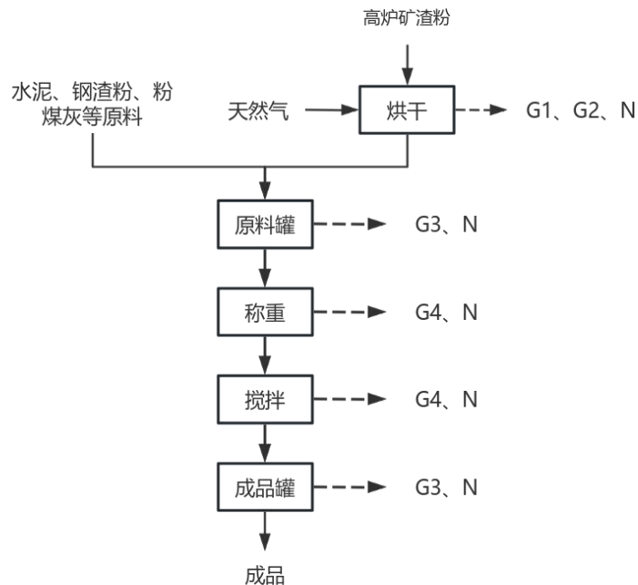
图 2-2 岩土固化剂生产工艺流程图
