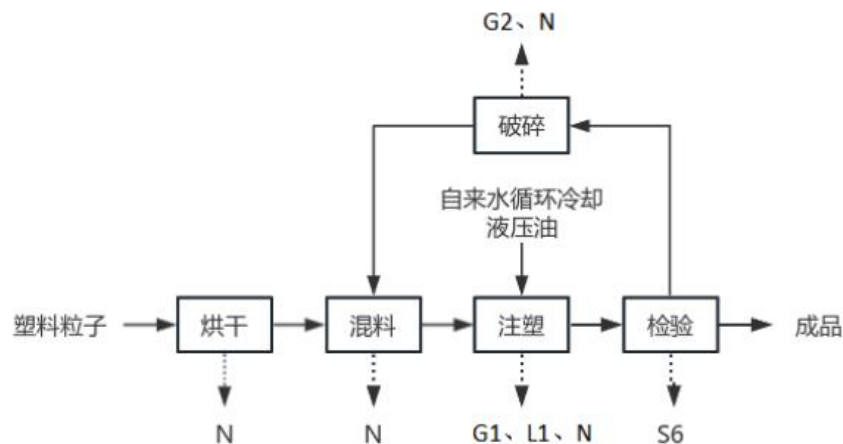
图 2-2 塑料制品加工工艺流程图
