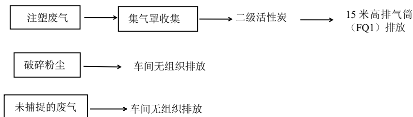
图 4-1 废气处理方式示意图
